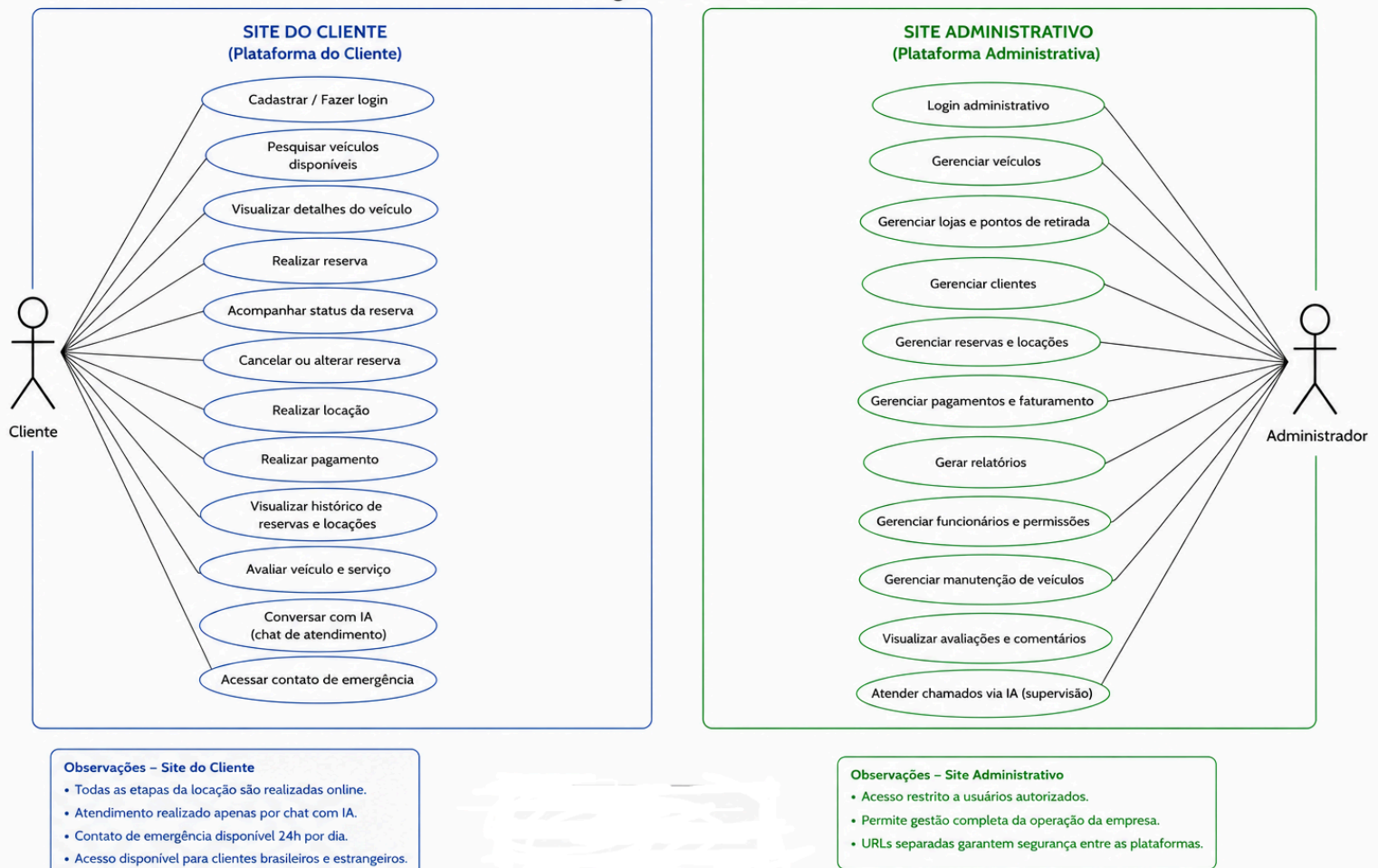
Diagrama de Caso de Uso
